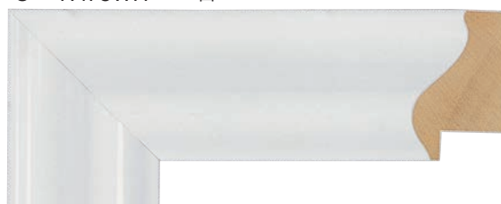
見え幅 47 / 幅 37 / カカリ 10 / 高さ 30 / 深さ 21
